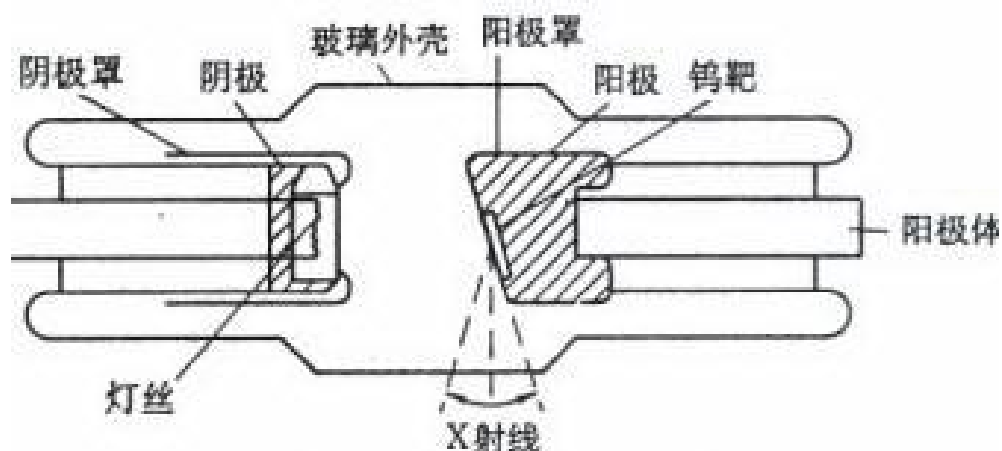
图 2-6 典型的 X 射线管结构示意图
