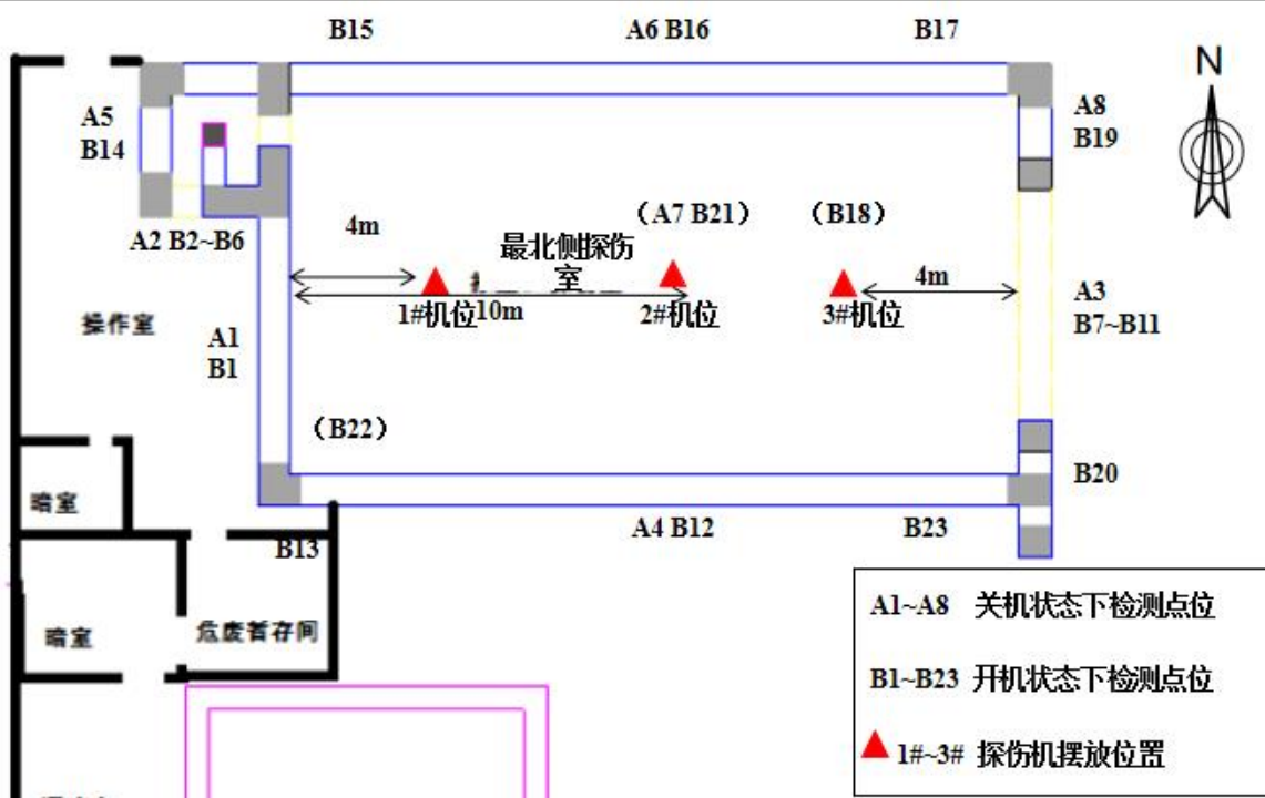
图 6-1 X-γ辐射剂量率检测布点示意图（XXGHZ-3505 型 X 射线探伤机）
